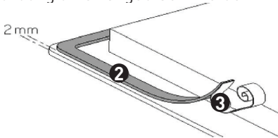
Dichtung ② nach Abnehmen der Schutzfolie in 2 mm Abstand vom äußeren Rand des Kochfelds aufkleben ③.
